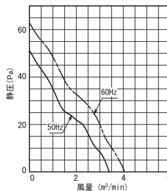
PF-155HL-M PF-155HL-2M
