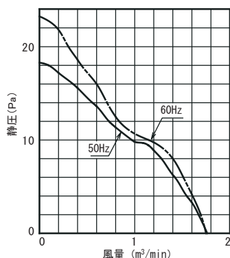
PF-125CHL-M PF-125CHL-2M
