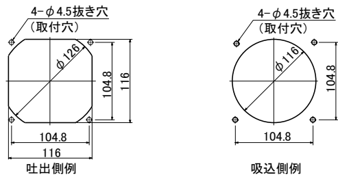
PF-125CHL-M、PF-125CHL-2M
