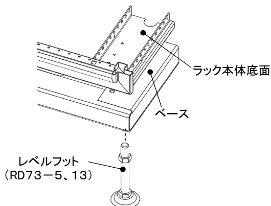
レベルフット取付部詳細図
