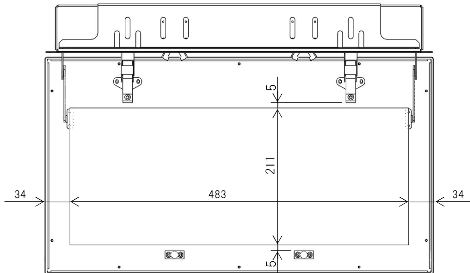
キーボード取付有効スペース
