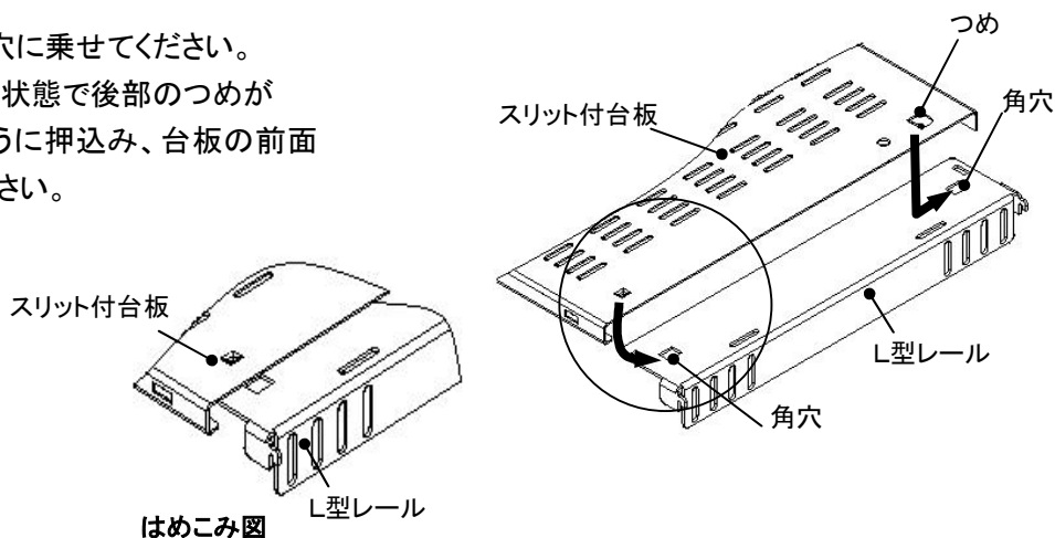
スリット付台板セット(RD152-□S)
