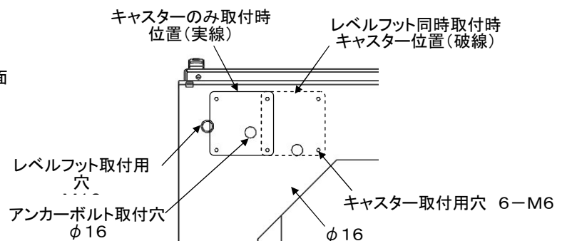
キャスター・レベルフット取付部詳細図
