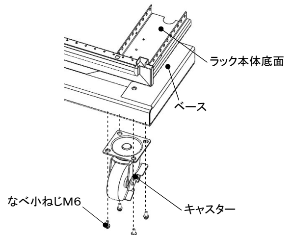
キャスター取付部詳細図
